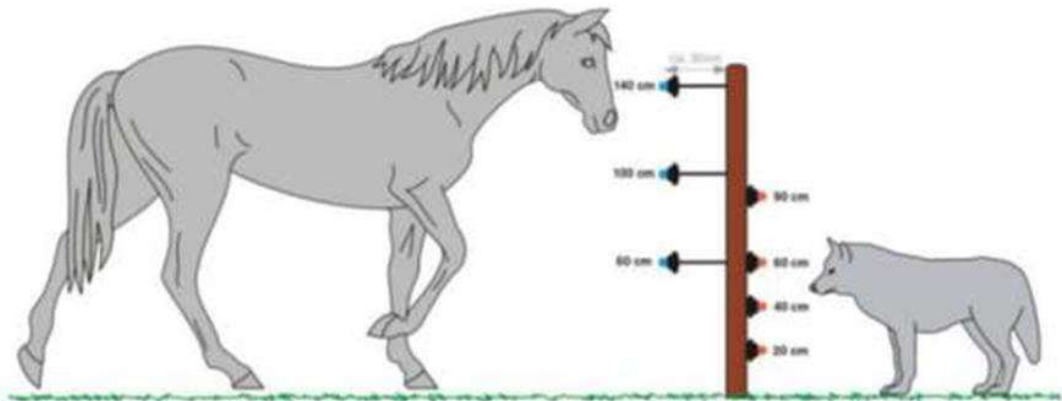
Binnenste draden op afstandhouders (tekening door G. Herkert)
